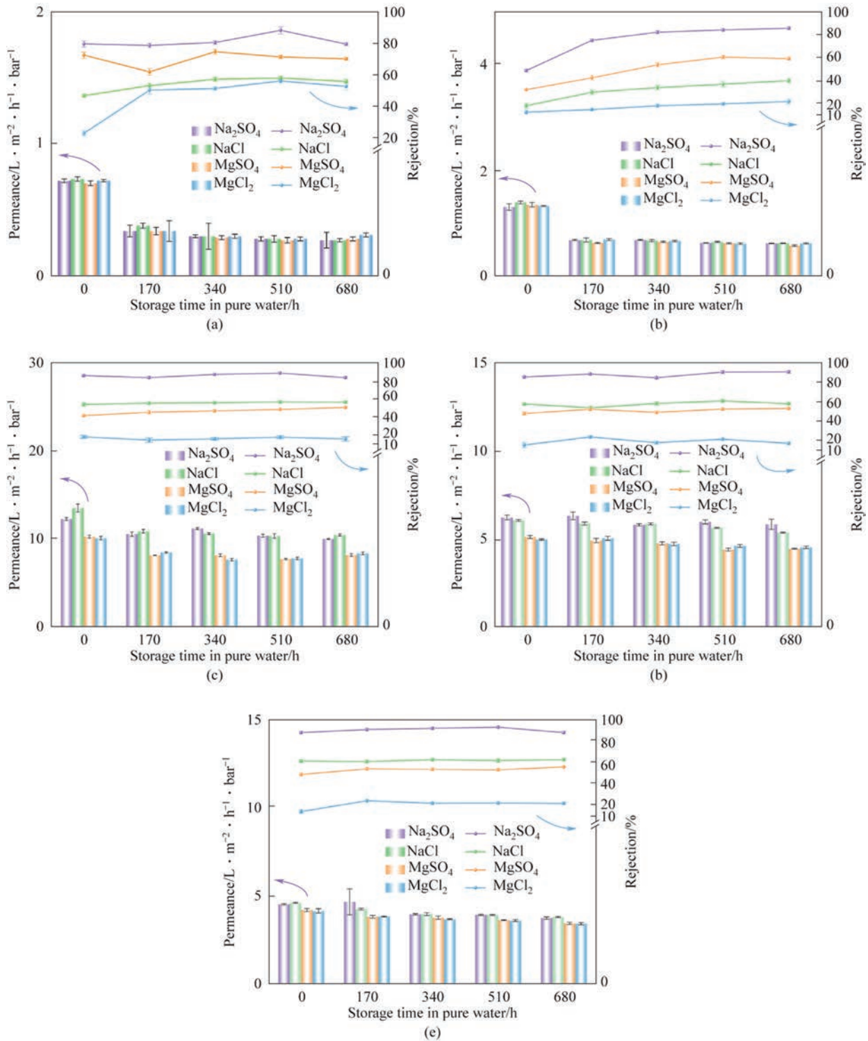
Fig. 14. Stability of GO and GE and PGE membranes (a) GO, (b) GE, (c) PGE-1, (d) PGE-2, (e) PGE-3.
